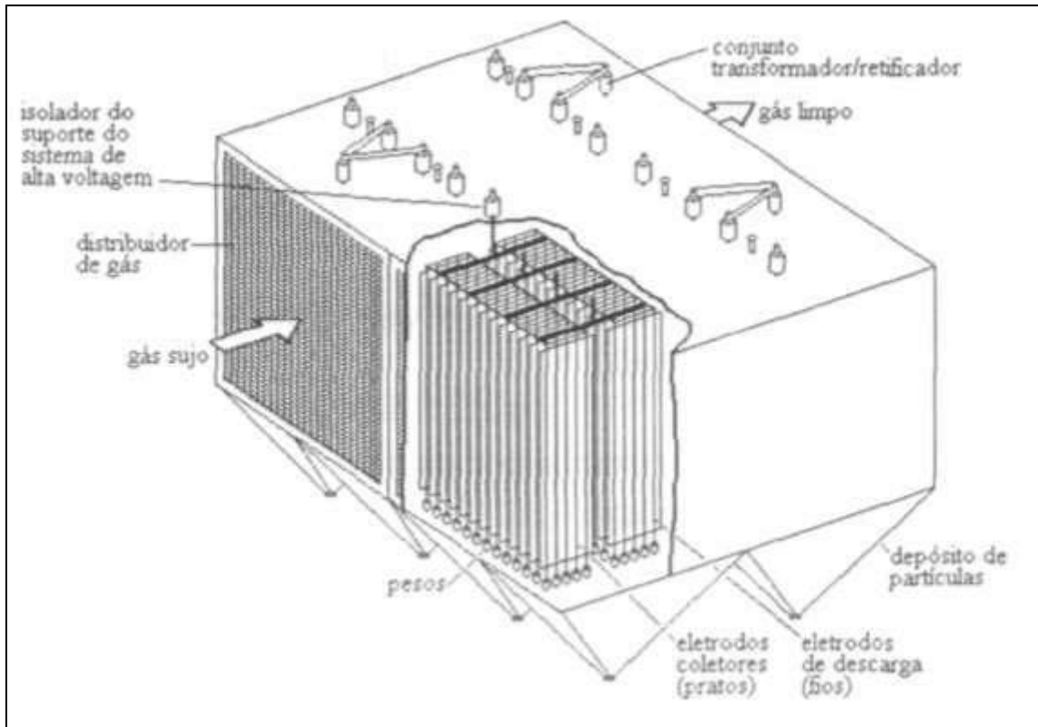
Figura 12 – Precipitador eletrostático
